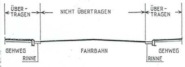
REGELQUERSCHNITT
